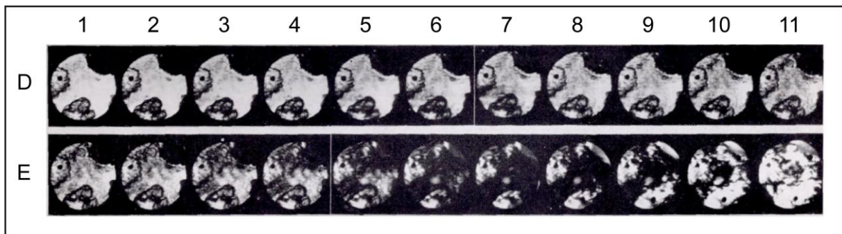
Bild 4.3: Ausschnitt aus einer Schlierenfotografiesequenz entnommen aus: NACA Report No. 912, 1948 /7/
