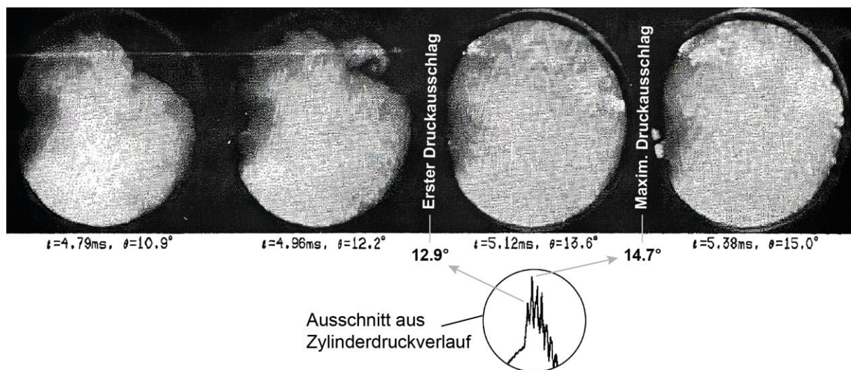
Bild 4.4: Eigenlichtaufnahmen vom Beginn eines Selbstzündungsvorgangs, entnommen aus Fig. 6 in /9/
